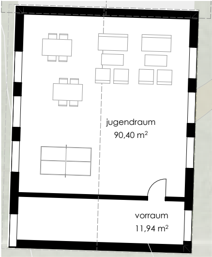
GRUNDRISS OG UMSPANNWERK
