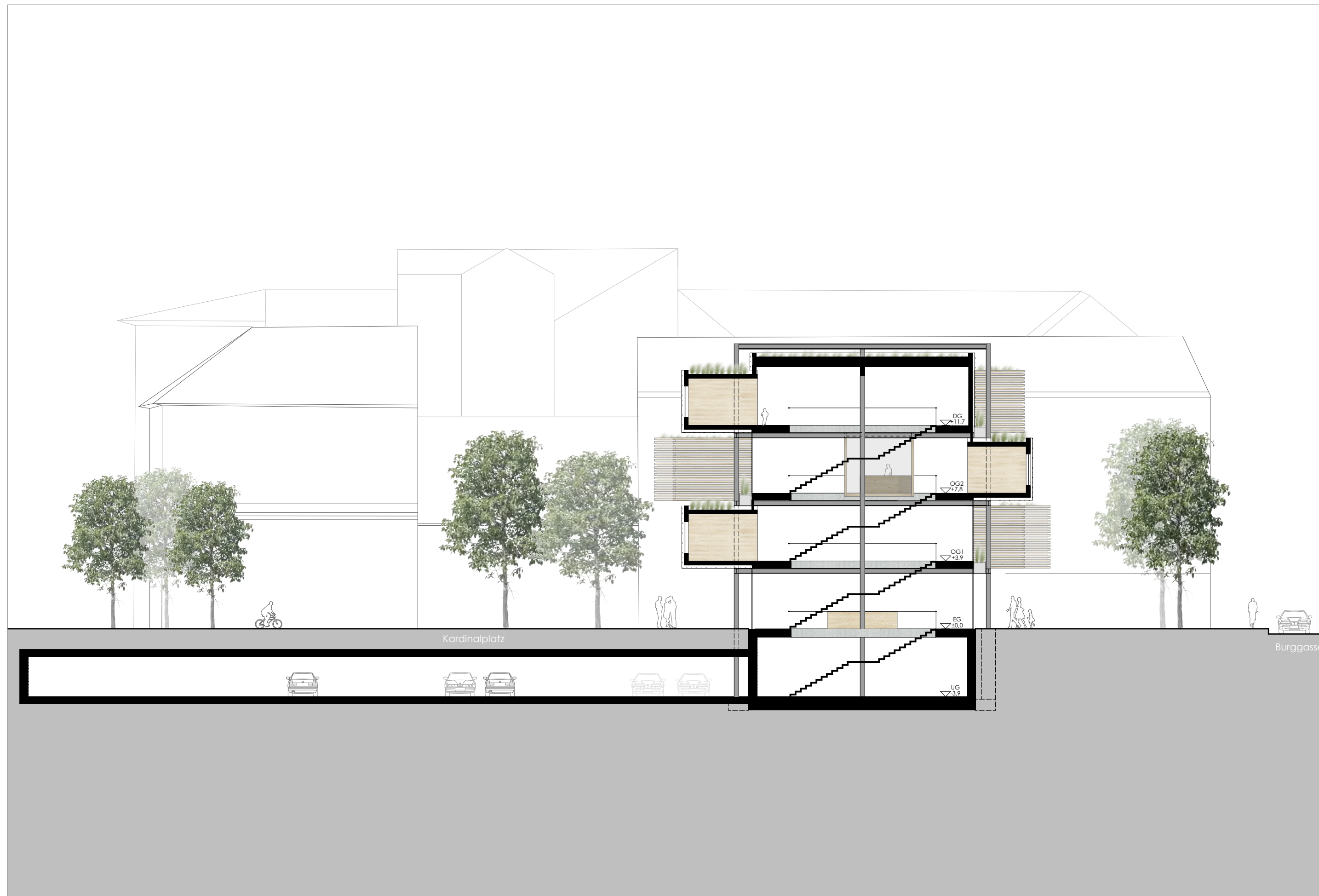
12 schnitt a-a
